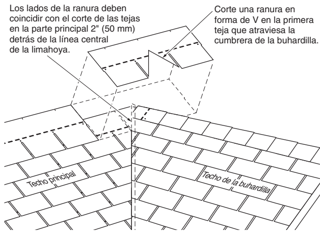
Figura 9-9: La teja con la ranura en V se ajusta sobre la cumbrera de la buhardilla.
