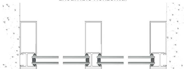
Ensamble Horizontal
