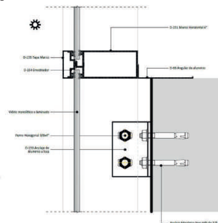
Sección vertical típica anclaje a losa
