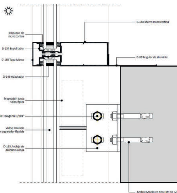
Sección vertical típica anclaje a losa
