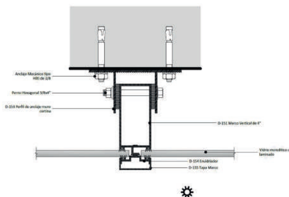
Sección horizontal típica anclaje a losa
